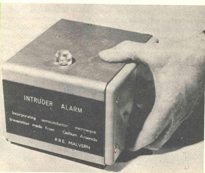
Fig. 3 - Sistema antifurto a microonde, realizzato dal Royal Radar Establishment.
