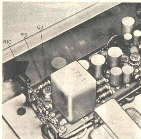
Si noti la disposizione del transistoro Q3 tipo 40407. Per i collegamenti della lampadina al neon PL1 è stata usata una basetta d'ancoraggio.
