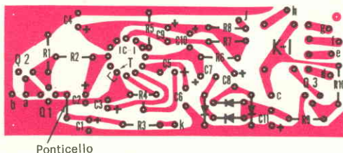
Fig. 3 - Disposizione dei componenti sul circuito stampato del rivelatore. Per Q1 occorre impiegare un normale zoccolo per transistori.
